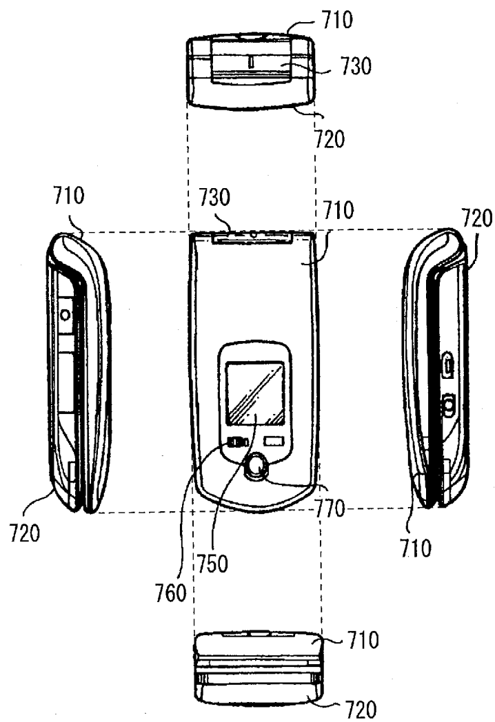
FIG. 19A
